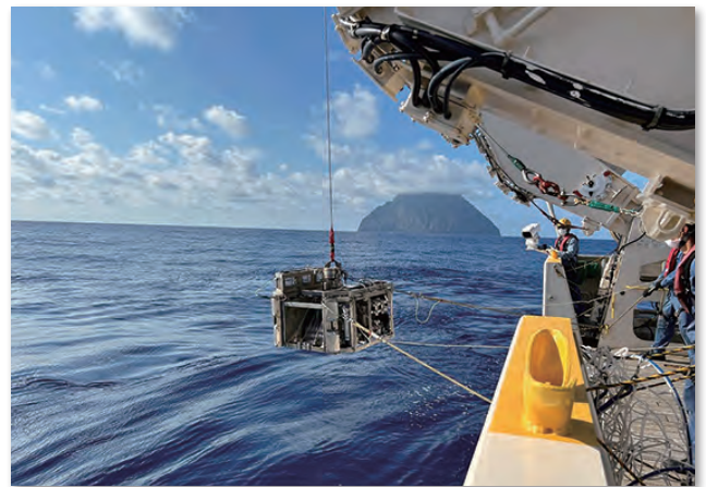
伊豆小笠原弧福徳岡ノ場火山における海底調査 Seafloor survey of the Fukutoku-Oka-no-Ba Volcano, Izu-Bonin Arc
