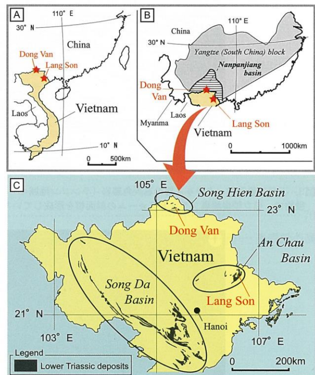
図1. A, 北部ベトナムにおける調査地域。B, 南中国ブロックに分布する下部三畳系ナンパンジャン海盆の古地理図 (Komatsu et al. , 2014を改訂)。C, アンチョウ, ソンヒエン, ソンダ堆積盆地の下部三畳系堆積物の分布。主な調査はドンバン地域やランソン地域で実施。
