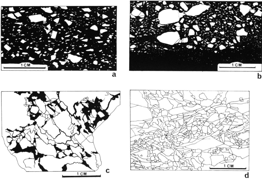
第8図. チャート角礫岩の組織. a: 泥質マトリックスの多い例, b: 泥質部との境界を示す例, c: 泥質マトリックスの少ない例で, チャート角礫どうしが縫合癒着している部分が認められる, d: 泥質マトリックスが全くない角礫化したチャート.
