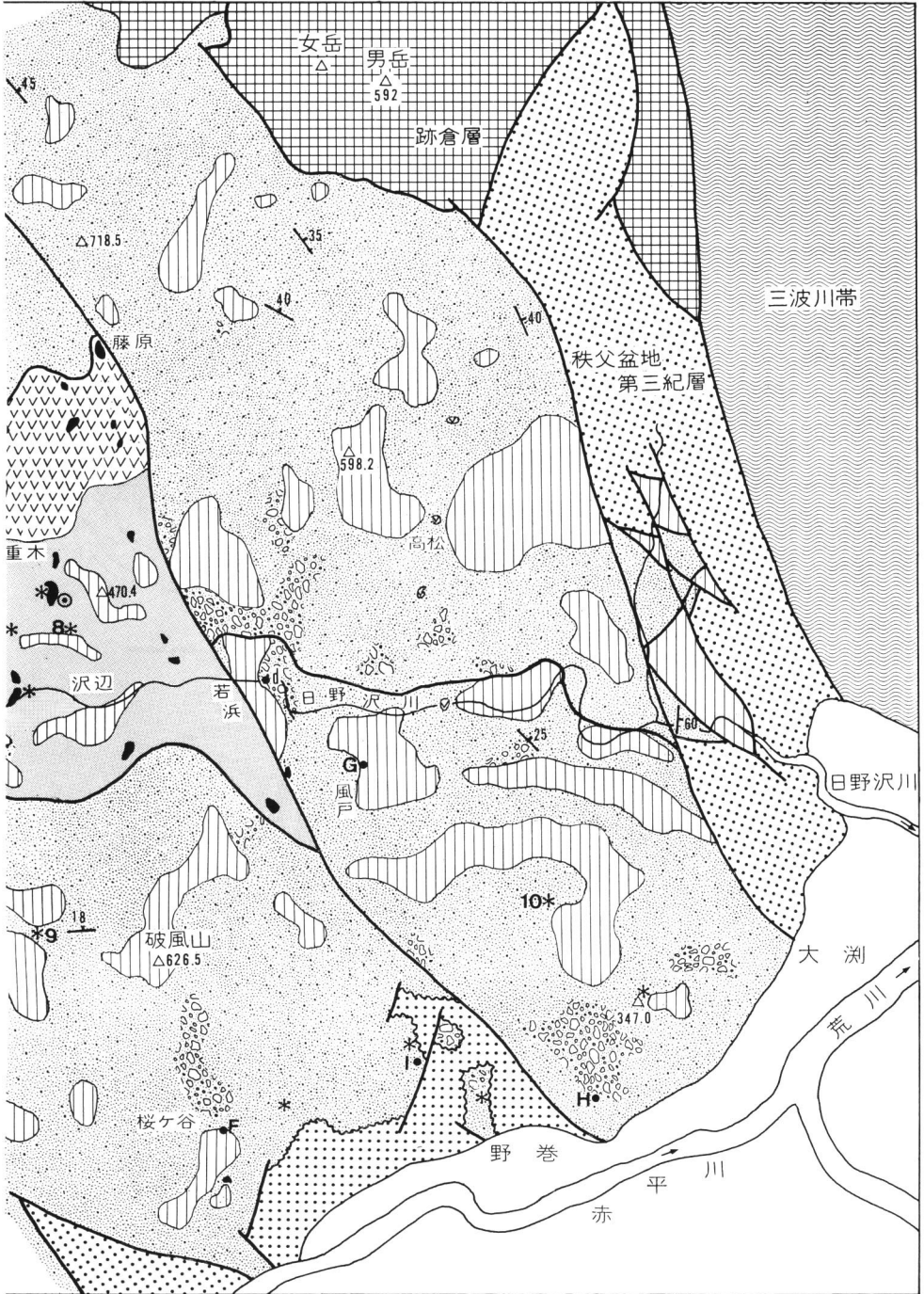
一ト・チャート角礫岩・緑色岩の産状を示すスケッチの位置，数字は放射虫化石の産出地点， 灰岩，7：緑色岩，8：放射虫化石産出地点，9：紡錘虫化石産出地点，10：断層
