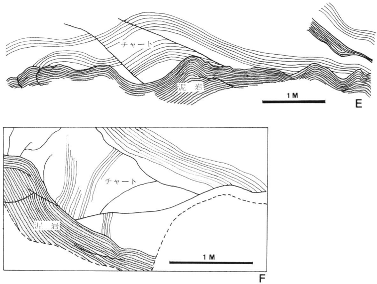
第5図. チャートの野外における産状. 一見整合にみえても, チャートの層理面が泥岩によって切られている例 (E 地点: 大前北方) と, チャートの層理面をほぼ直交して切る泥岩の例 (F 地点: 桜ヶ谷).
