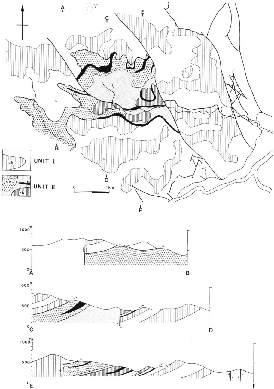
第3図. ユニット I とユニット II の分布を示す構造図および両者の関係を示す構造断面図. ch: チャート, ls: 石灰岩, gs: 緑色岩
