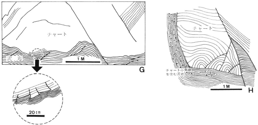
第6図. チャートの野外の産状. 小断層でずれているチャート (G 地点: 風戸) と小褶曲したチャート (H 地点: 野巻) のブロックをとりまく泥岩.
