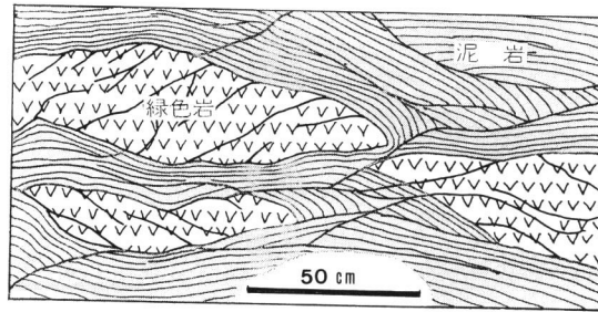
第9図. 緑色岩の産状例 (J 地点: 門平北西方).
