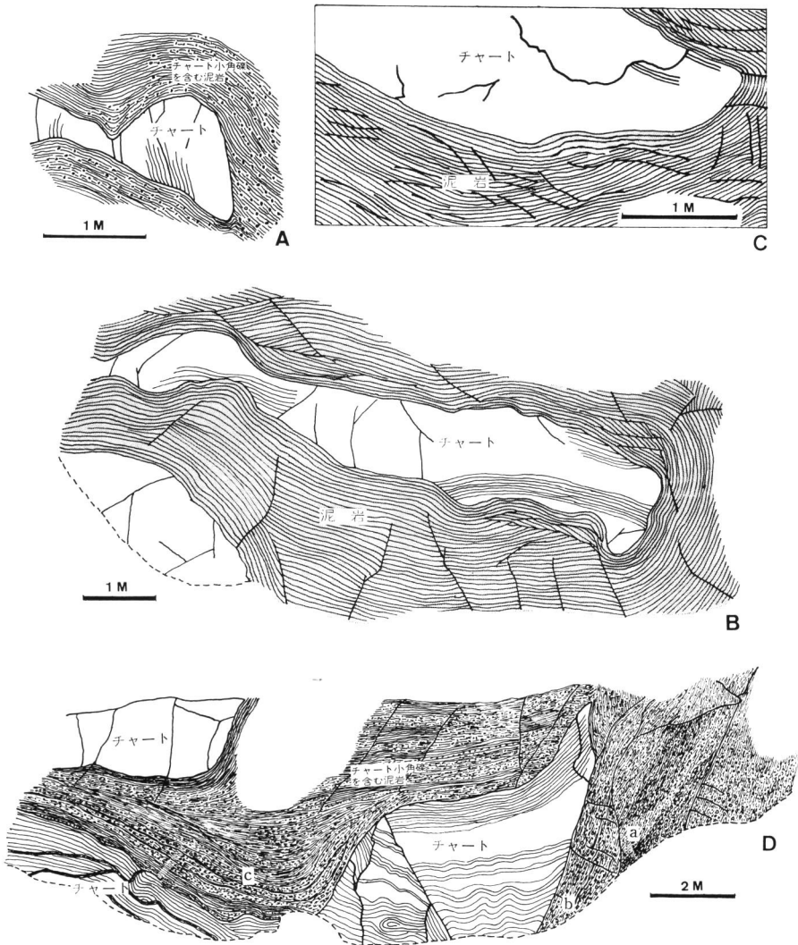
第4図. チャートの野外における産状. チャートの層理面を切って泥岩あるいはチャートの小角礫を含む泥岩がとりまいている例を示す (A, B, C および D 地点: 調査地北東部の城峰林道沿い, 地質図参照).
