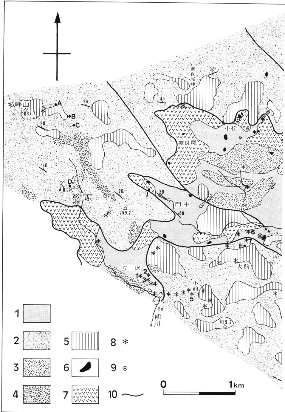
第2図. 関東山地北東部・埼玉県秩父日野沢地域の秩父累帯北帯の地質図。アルファベットはチャ 1: 泥岩, 2: 砂岩・砂岩泥岩互層, 3: 珪質凝灰岩, 4: チャート角礫岩, 5: チャート, 6: 石
