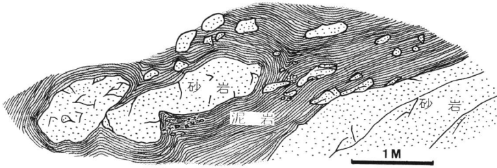
第7図. 砂岩の野外における産状例 (I地点: 野巻北西).
