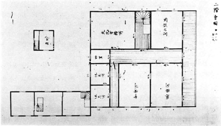
図 4 第 1, 2 回目二階, 物見平面図 (計画案)
