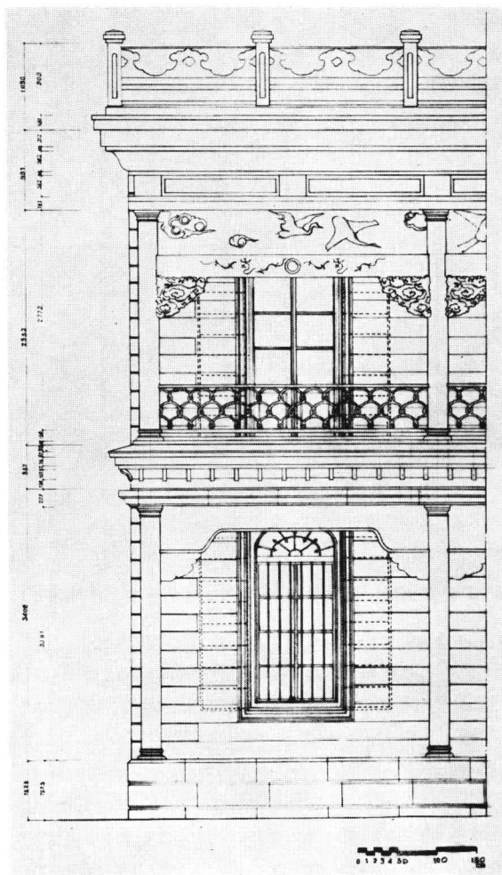
図 7 正面詳細図
