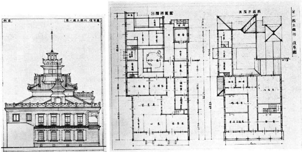
図 2 堀越三郎復元図
