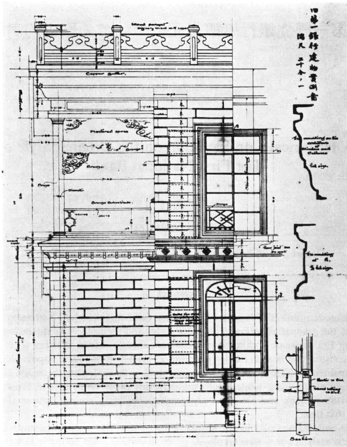
図 1 森山松之助実測詳細図
