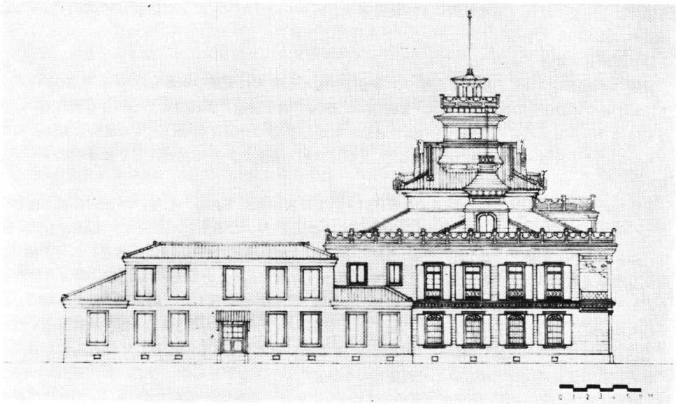
図 8 側面図 (正面に向き左側面). なお正面は堀越復元案に準じ略す
