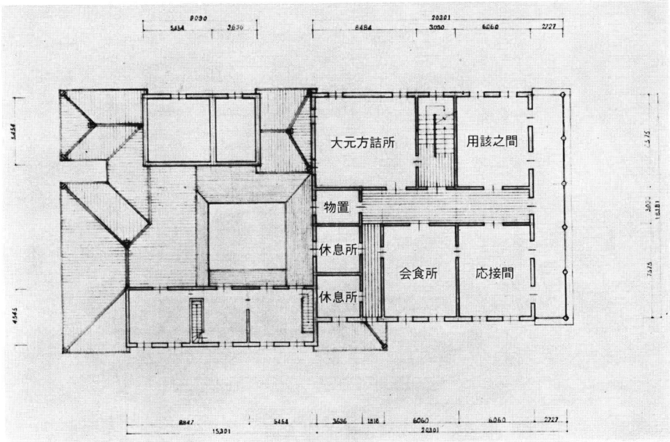
図 6 2 階平面図・屋根伏図。(室名は「計画案」を参考にした)
