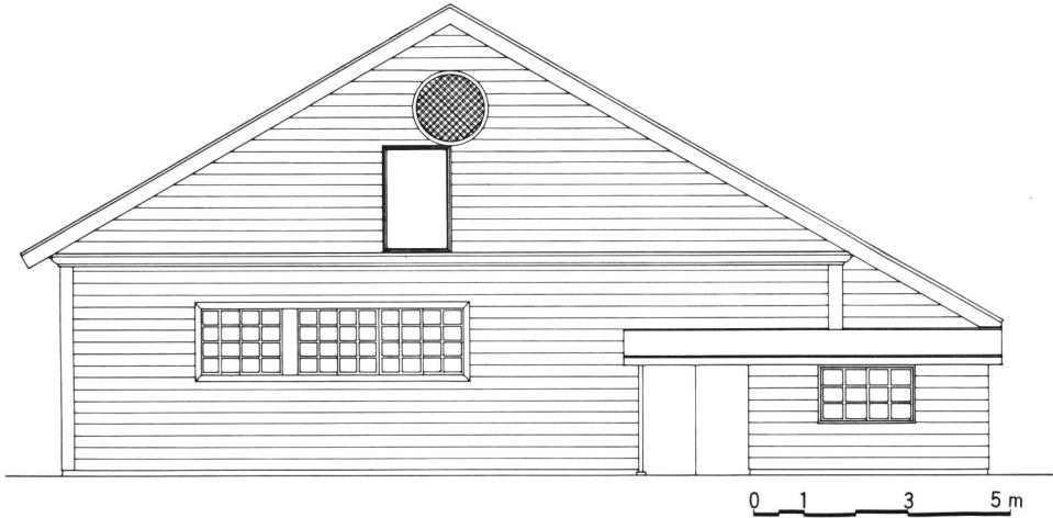
図 14 旧紬糸工場東側実測立面図
