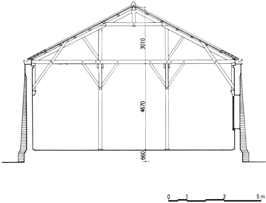
図 12 旧製品倉庫実測断面図
