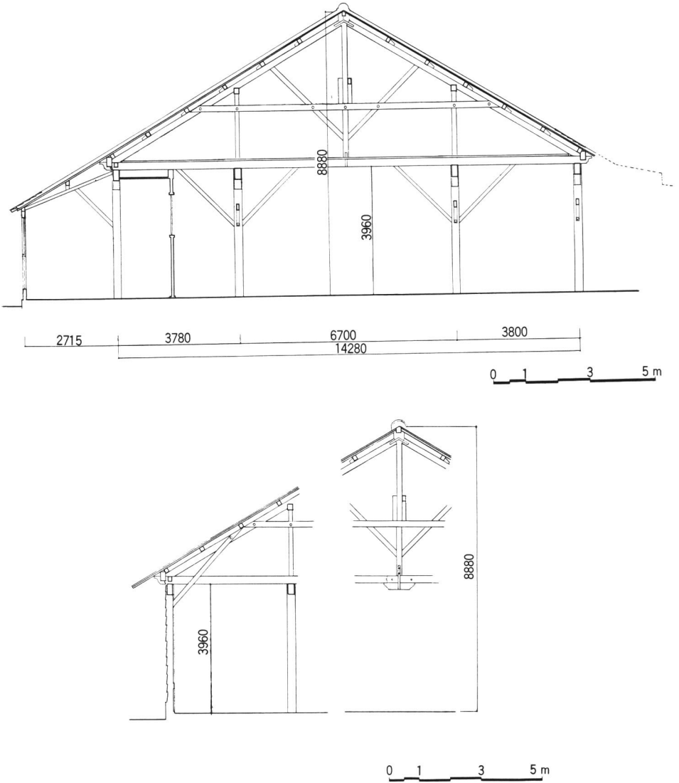
図 13 旧細糸工場実測断面図
