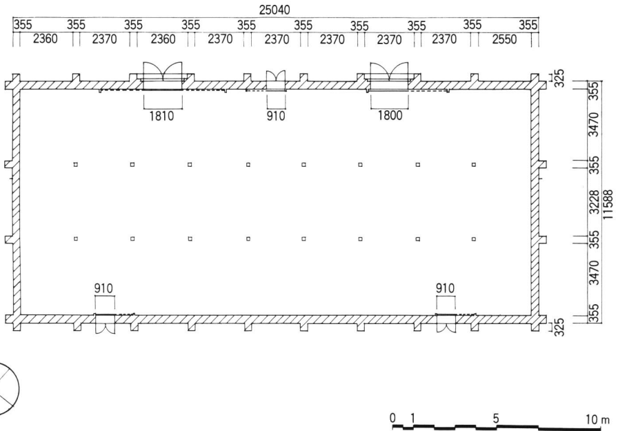
図 11 旧製品倉庫実測平面図
