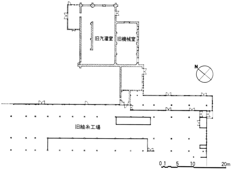
図 10 旧汽灌室・旧機械室・旧糸工場 (一部) 実測平面図
