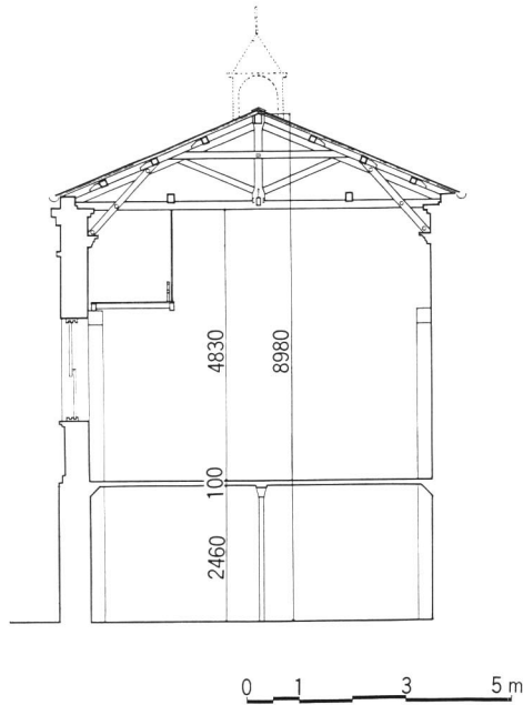
図 8 旧機械室実測断面図
