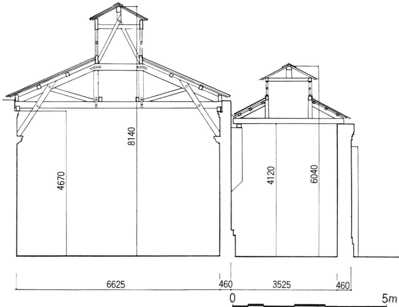
図 7 旧汽灌室実測断面図
