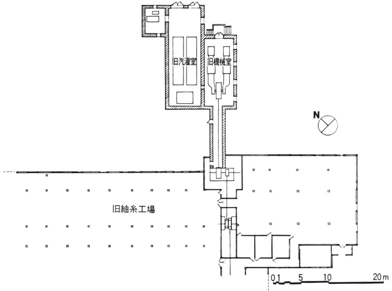
図 9 鐘紡合併時頃の平面図 (原図を部分トレースしたもの)
