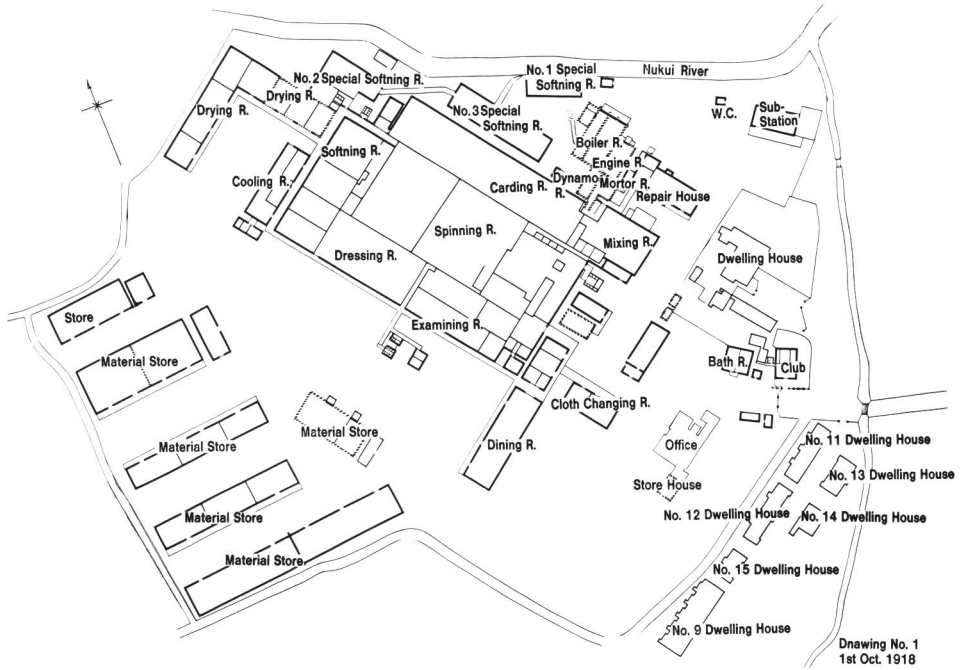
図 4 大正 7 年の平面図 (“KANEGAFUCHI SPINNING COMPANY LTD. SHIMMACHI SILK MILL” よりトレース。主要な施設名のみ記入, R は Room の略記)
