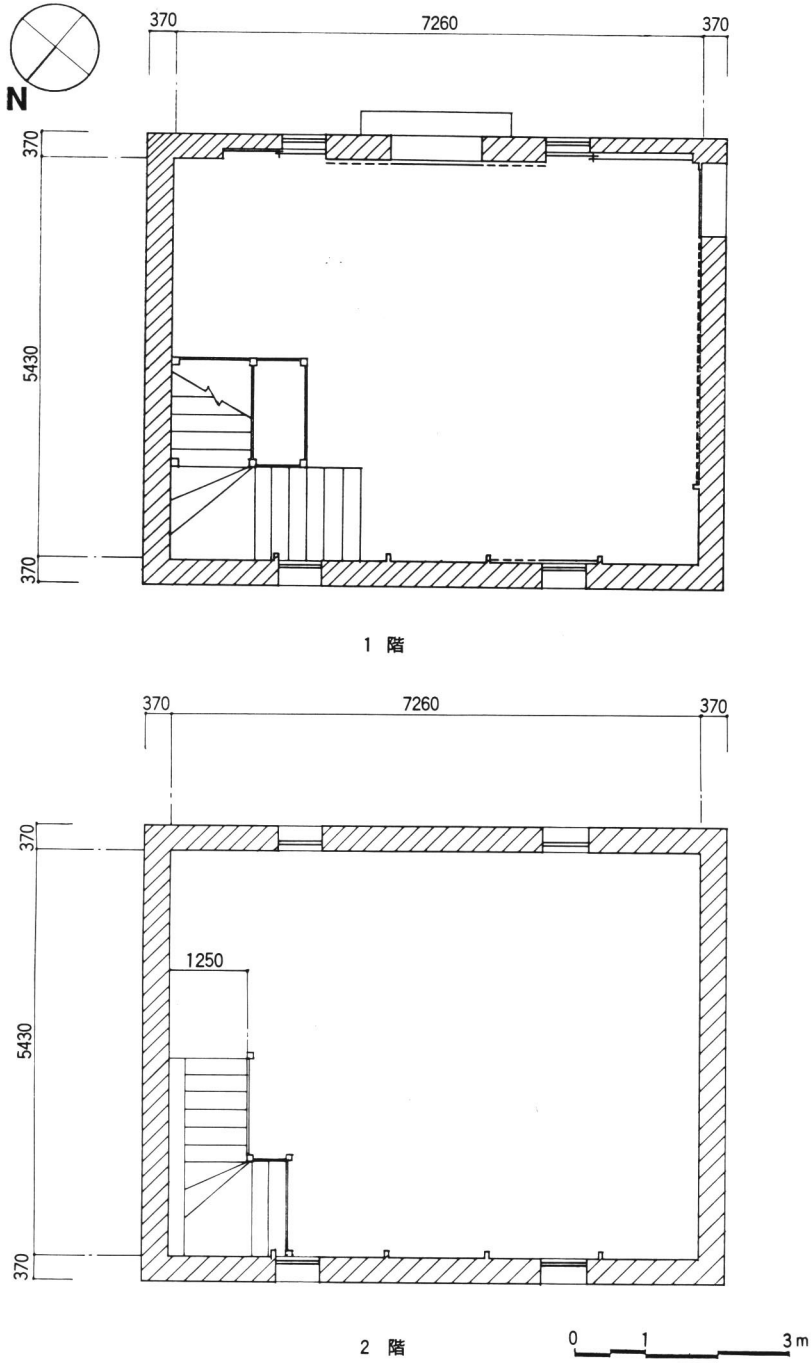
図 6 旧二階家煉瓦庫実測平面図
