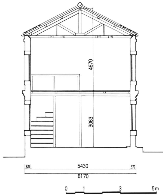
図 5 旧二階家煉瓦庫実測断面図
