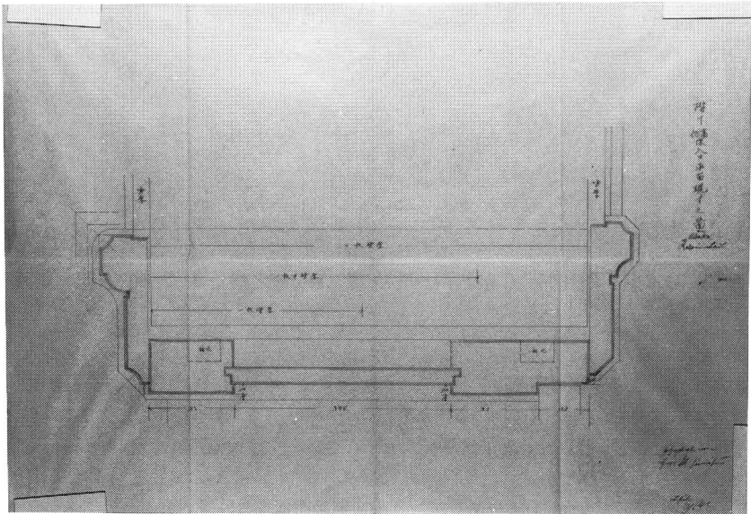
写真 30 大阪控訴院図面（「階下高低床入口平面原寸之圖」, 80.0×55.5(cm), 美濃紙, 鉛筆一部彩色, 日付不明）
