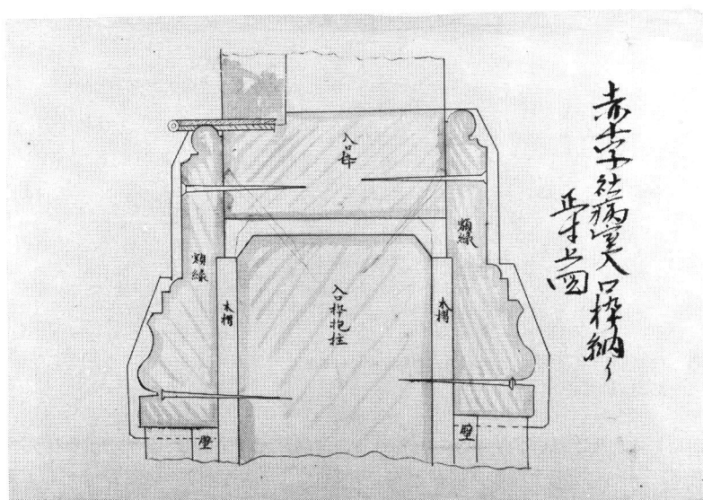
写真 7 日本赤十字社図面（「赤十字社病室入口棹納り正寸上図」, 39.0×27.3(cm), 美濃紙, 墨入り彩色一部鉛筆, 日付不明）
