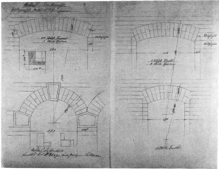
写真 12 東京裁判所図面（「Neubaw: Saibansho Kellergeschos Fenster der Hof」, 41.0×32.5 (cm), 鉛筆, 日付不明）
