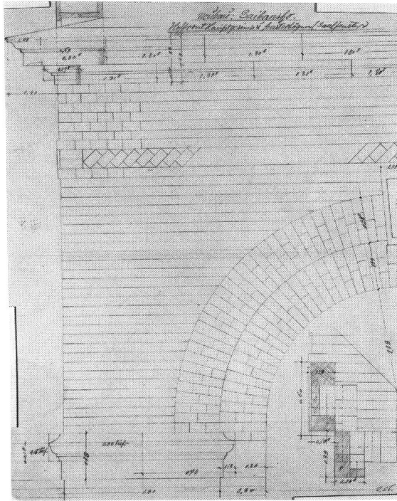
写真 23 東京裁判所図面 (「Neubau: Saibansho. Hoffront Hauptgesimse u Feusterbogrer (Saalfauster)」, 32.5×41.3(cm), 美濃紙, 鉛筆, 日付不明)
