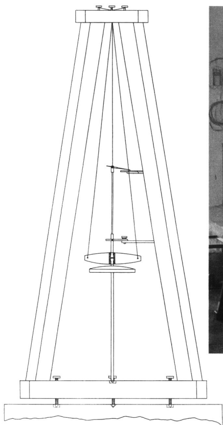
第2図 簡単地震計
